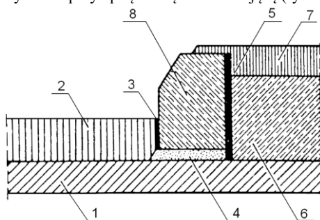
Rys. 4.1. Przykład wykonania krawężnika: 1- warstwa wiążąca, 2 - warstwa ścieralna, 3 - samoprzylepna taśma uszczelniająca połączenie warstwy ścieralnej z krawężnikiem, 4 - masa zalewowa w złączeniu podłużnym, 5 - masa zalewowa w złączeniu poprzecznym, 6 - płyta betonowa, 7 - warstwa ścieralna z asfaltu lanego na chodniku, 8 - krawężnik kamienny
