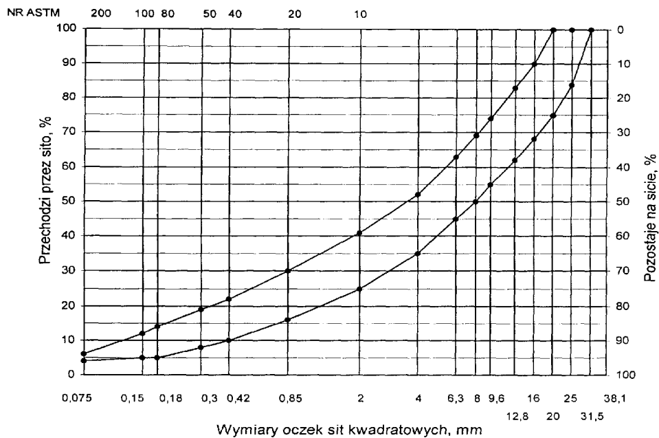
Rys. 12. Krzywe graniczne uziarnienia mieszanki mineralnej BA od 0 do 20 mm do warstwy wiążącej, wyrównawczej i wzmacniającej nawierzchni drogi o obciążeniu ruchem od KR3 do
