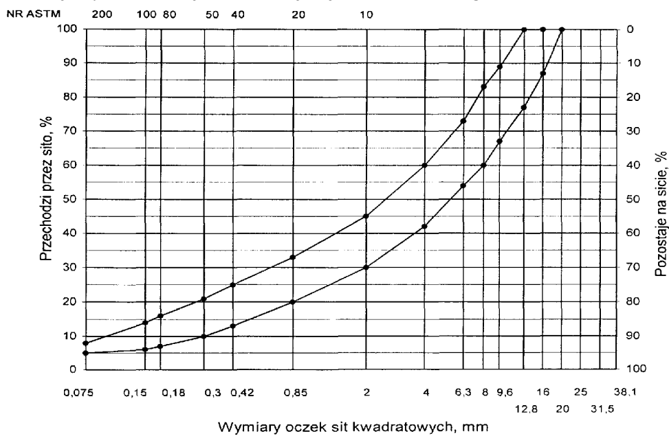
Rys. 12. Krzywe graniczne uziarnienia mieszanki mineralnej BA od 0 do 20 mm do warstwy wiążącej, wyrównawczej i wzmacniającej nawierzchni drogi o obciążeniu ruchem od KR3 do
